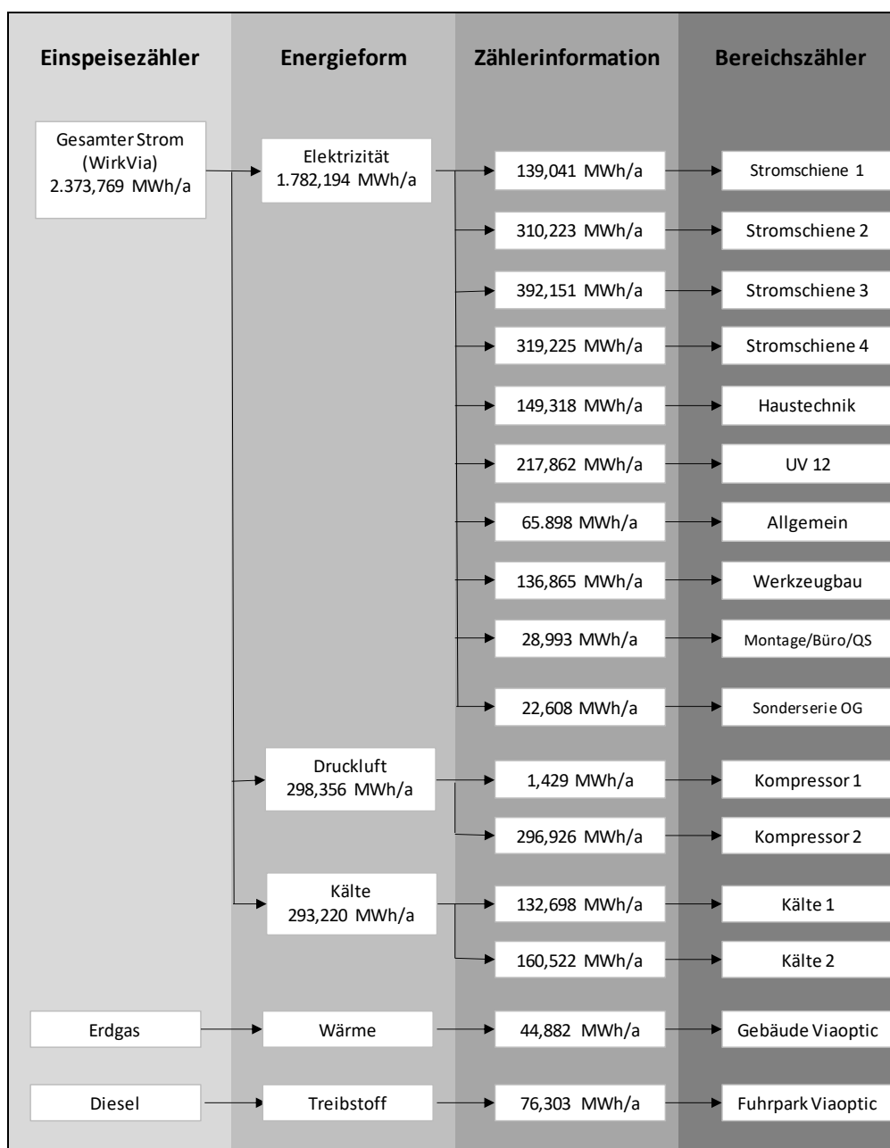
Abbildung 7: Energieanalyse 2023 der VIAOPTIC GmbH
