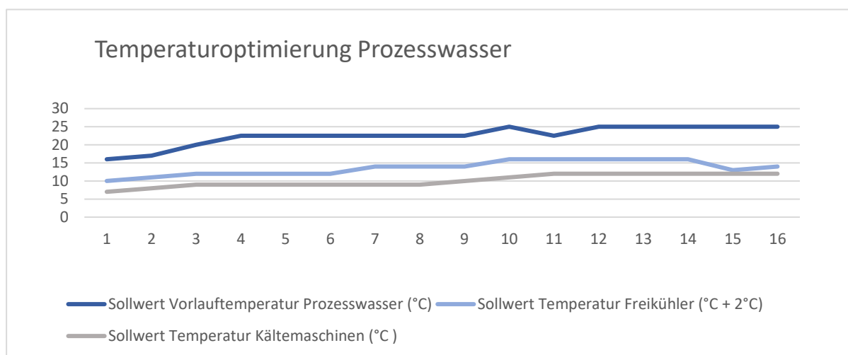
Abbildung 9: Temperaturoptimierung Prozesswasser
